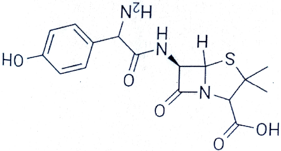
Amoxicillin
