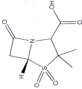
Sulbactam
