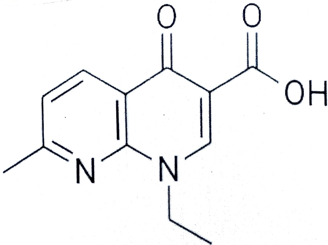
Nalidixic acid
