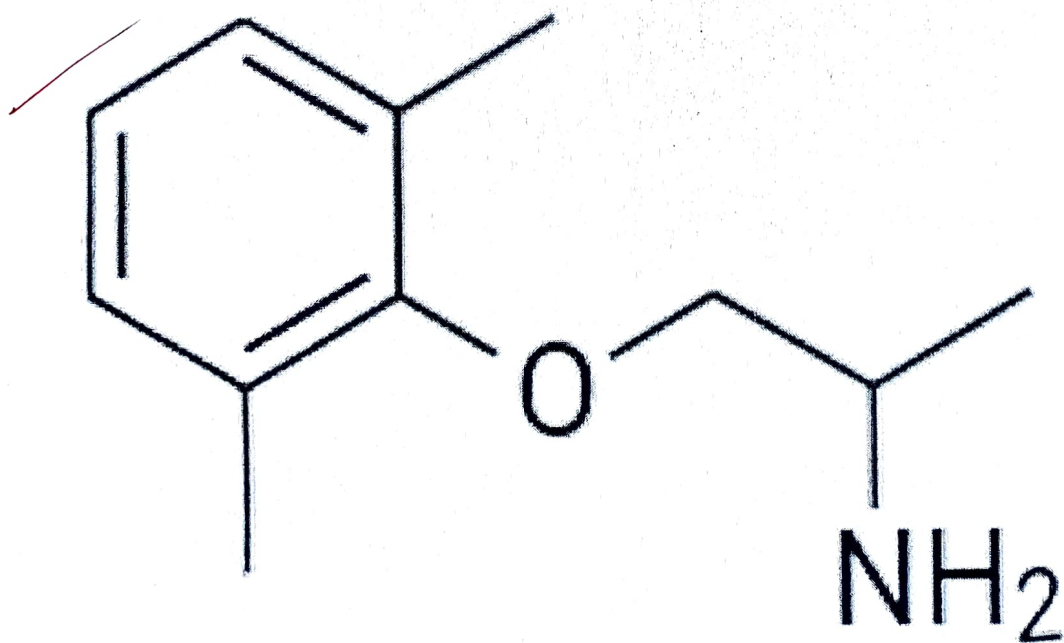
Mexiletine
